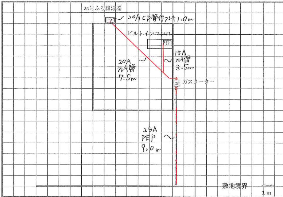
内管工事見積用平面図
